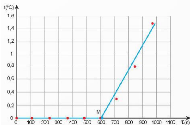
Hình 5.1. Đồ thị biểu diễn sự thay đổi nhiệt độ theo thời gian của nước trong bình nhiệt lượng kế từ số liệu Bảng 5.2
