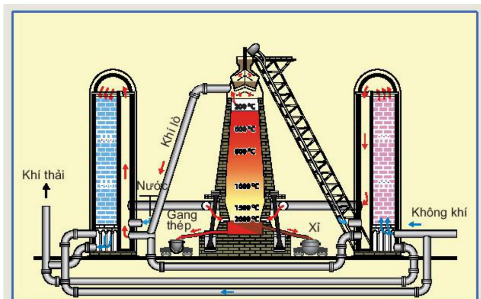
Hình 3.2. Sản xuất gang – thép trong lò cao (SGK tr.14)
