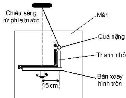
Hình 4.2. Con lắc đơn dao động điều hòa
