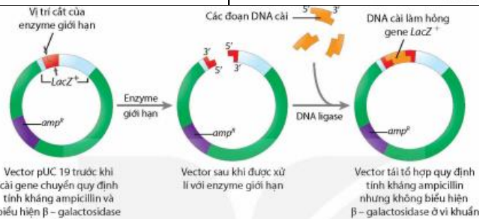
Hình 3.5. Phương pháp cài đoạn DNA đích vào vector
