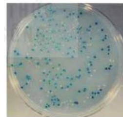
Hình 3.4. Phương pháp chọn lọc khuẩn lạc xanh – trắng khi sử dụng vector pUC19 Các khuẩn lạc mọc trên môi trường chứa ampicillin là các khuẩn lạc chứa vector (nhỏ có gene amp r ); các khuẩn lạc xanh không mang gene cải nên gene lacZ + còn nguyên vẹn (enzyme này chuyển hoá X-gal thành chất có màu xanh). Các khuẩn lạc trắng gồm các tế bào mang gene đích đã được cài vào vector
