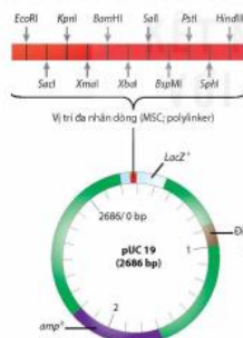
Hình 3.3. Vector nhân dòng plasmid pUC19 Ori = trình tự khởi đầu tái bản, amp r = gene chỉ thị chọn lọc kháng kháng sinh ampicillin, lacZ + = gene chỉ thị chọn lọc mã hoá \beta - galactosidase
