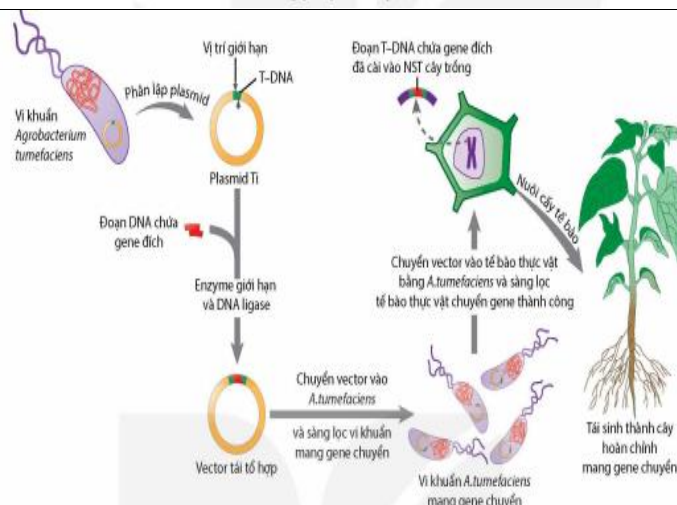
Hình 3.6. Các bước chuyển gene ở cây trồng sử dụng vector plasmid Ti và vi khuẩn Agrobacterium tumefaciens
