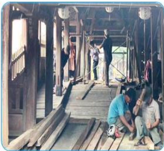
Hình 3.1. Chùa Cầu (Hội An) đang được chống đỡ
