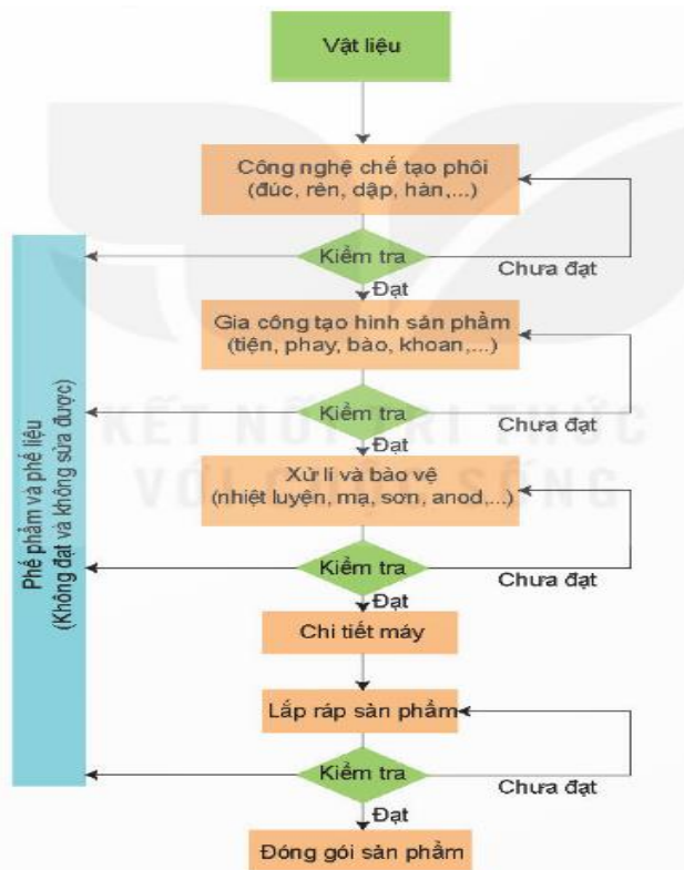
Hình 11.2. Quá trình sản xuất cơ khí
